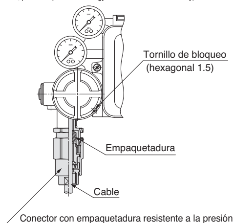
Prensaestopas con empaquetadura resistente a la presión (opcional)
