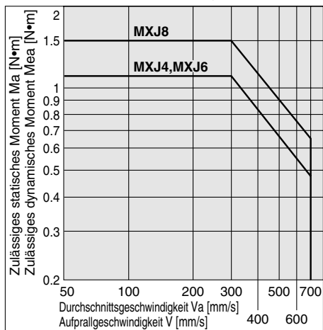
Grafik (2) Zulässiges Moment Längsbelastung: M_{ap} , M_{ep} Querbelastung: M_{ay} , M_{ey}
