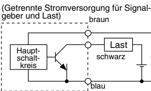
Spezifizierung für Anschluss an SPS mit COMMON Plus
