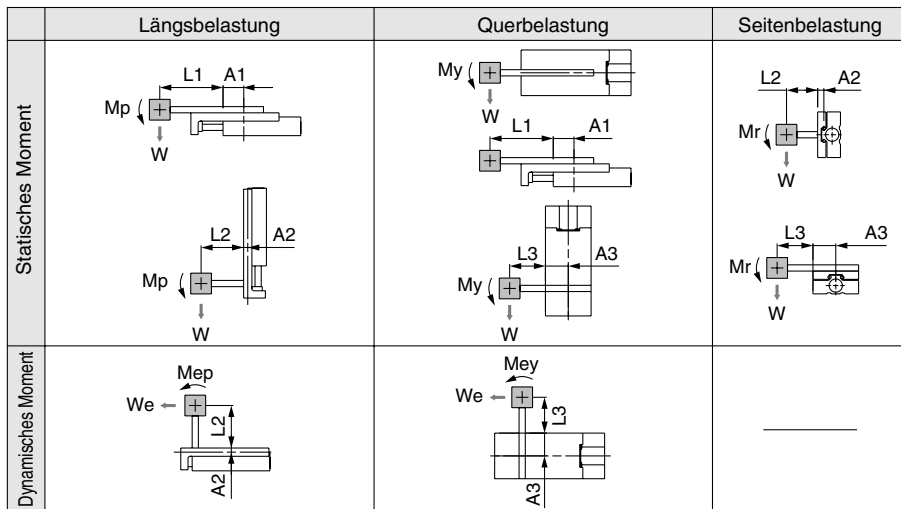
Abb. (1) Überstand: L_n [mm], Korrekturwert für Abstand Tisch-Lastdrehpunkt: A_n [mm]
