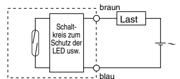
2-Draht-System <Reedkontakt-Signalgeber>
