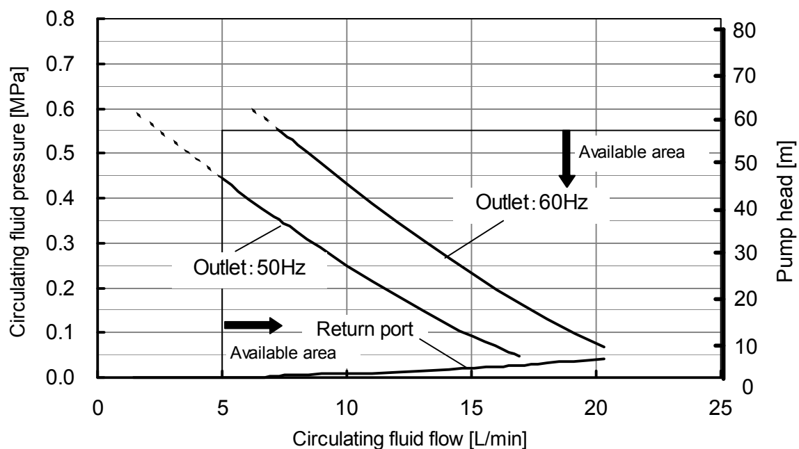
Fig. 9-16 Pump capacity(HRS012-**-10-T, HRS018-**-10-T, HRS012-**-10-MT, HRS018-**-10-MT)
