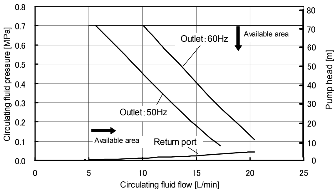
Fig. 9-17 Pump capacity(HRS012-**-20-T, HRS018-**-20-T, HRS024-**-20-T)
