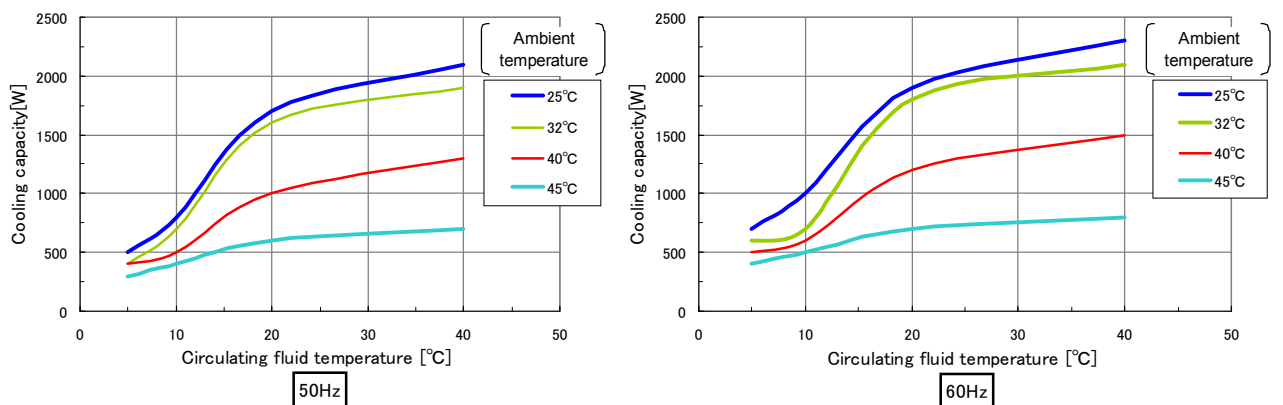
Fig. 9-10 Cooling capacity (HRS018-A*-20-G)
