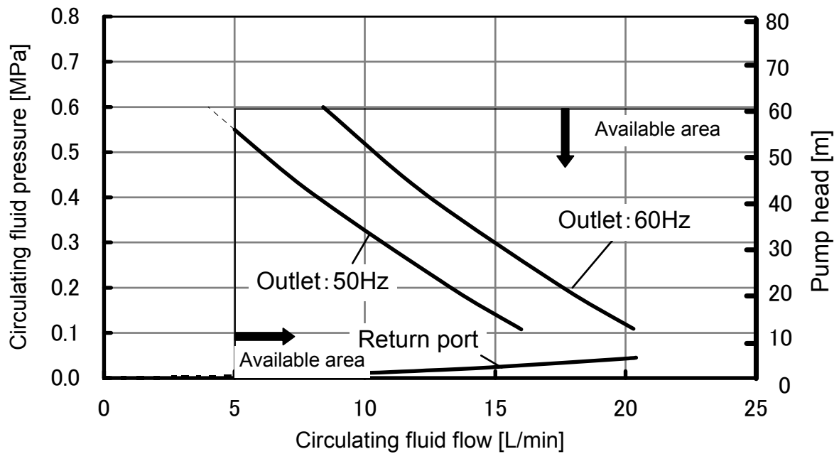
Fig. 9-18 Pump capacity(HRS012-**-20-MT, HRS018-**-20-M, HRS024-**-20-MT)
