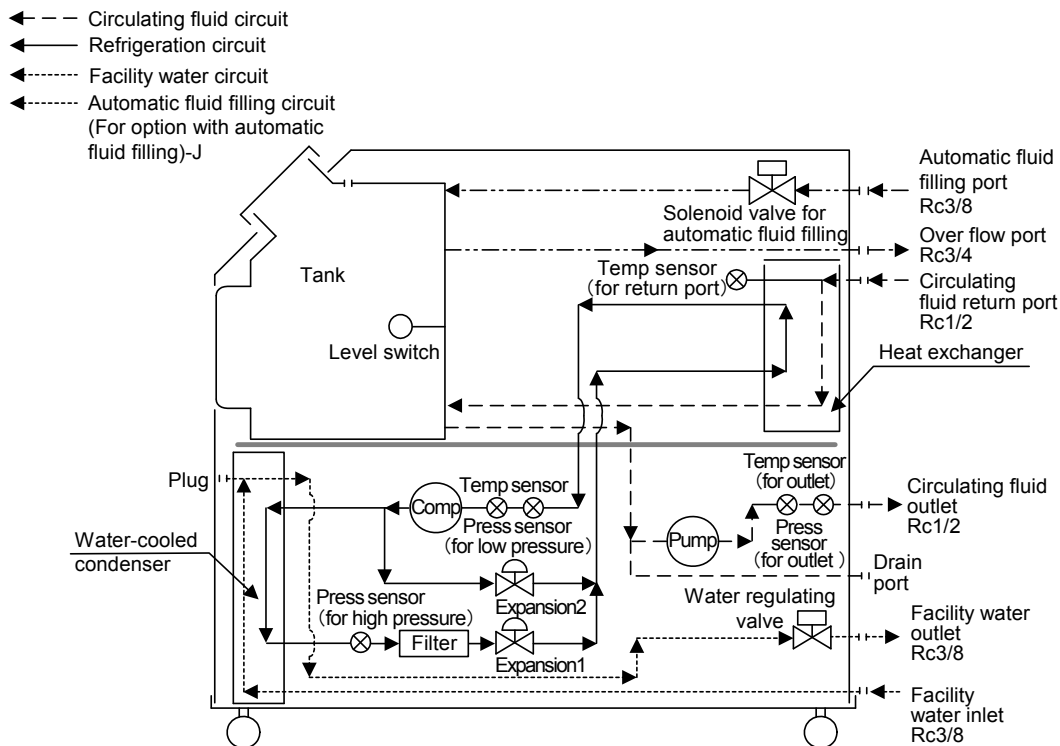
Fig. 9-3 Flow Chart(HRS012-W*-0, HRS018-W*-0, HRS024-W*-20)
