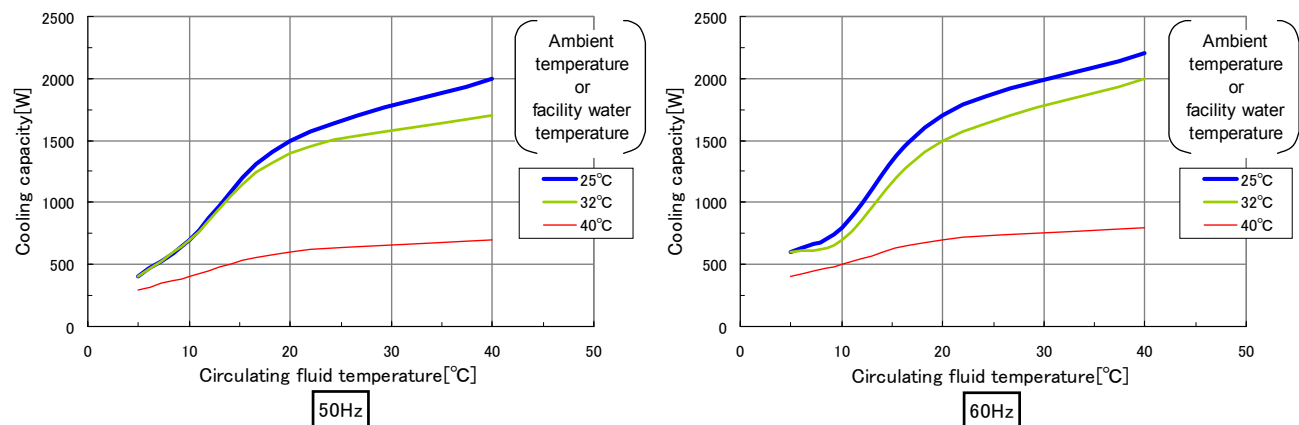
Fig. 9-5 Cooling capacity(HRS018-**-10)
