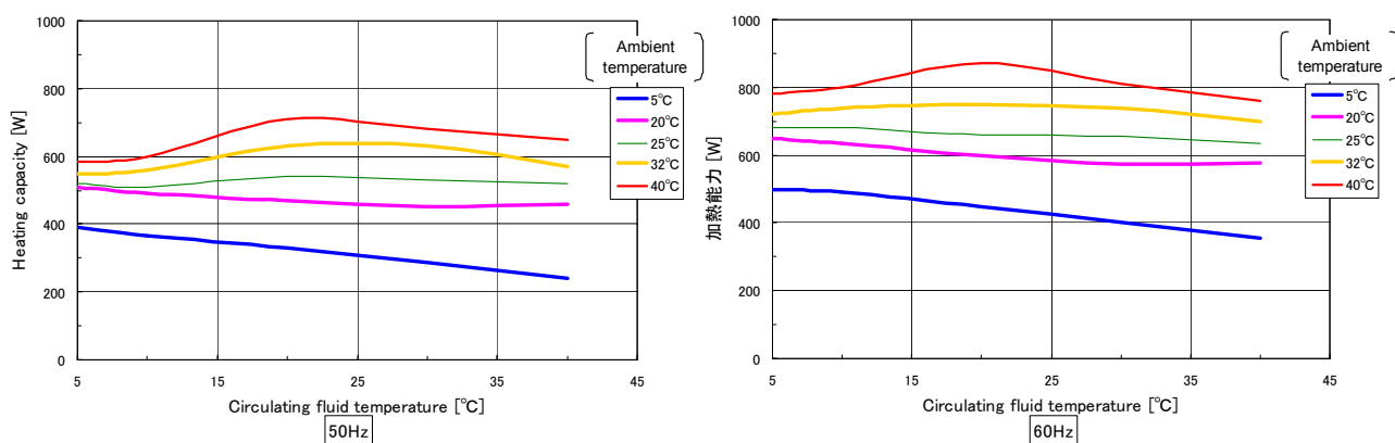
Fig. 9-13 Heating capacity(HRS012-**-20, HRS018-**-20, HRS024-**-20)
