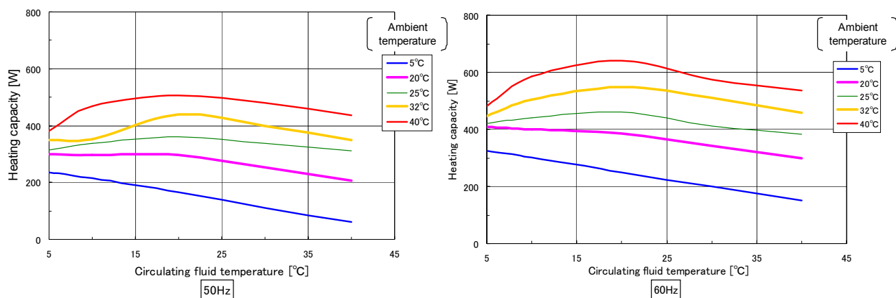
Fig. 9-12 Heating capacity(HRS012-**-10, HRS018-**-10)
