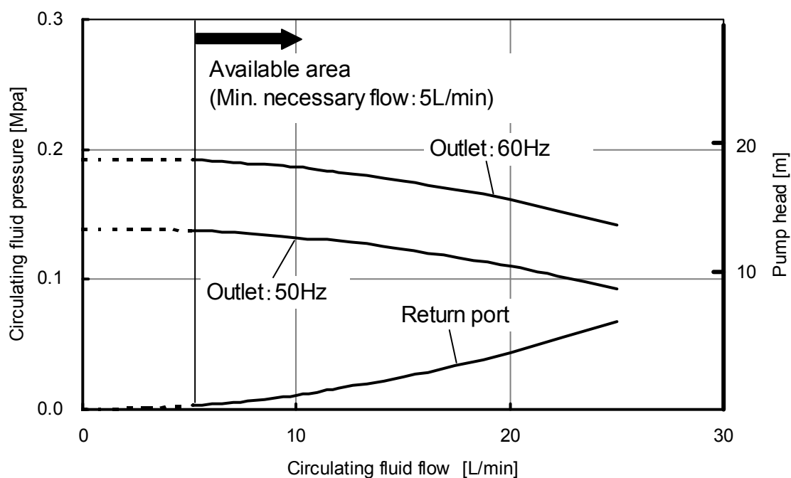
Fig. 9-15 Pump capacity(HRS012-**-20-(BGJM), HRS018-**-20-(BGJM), HRS024-**-20-(BGJM))
