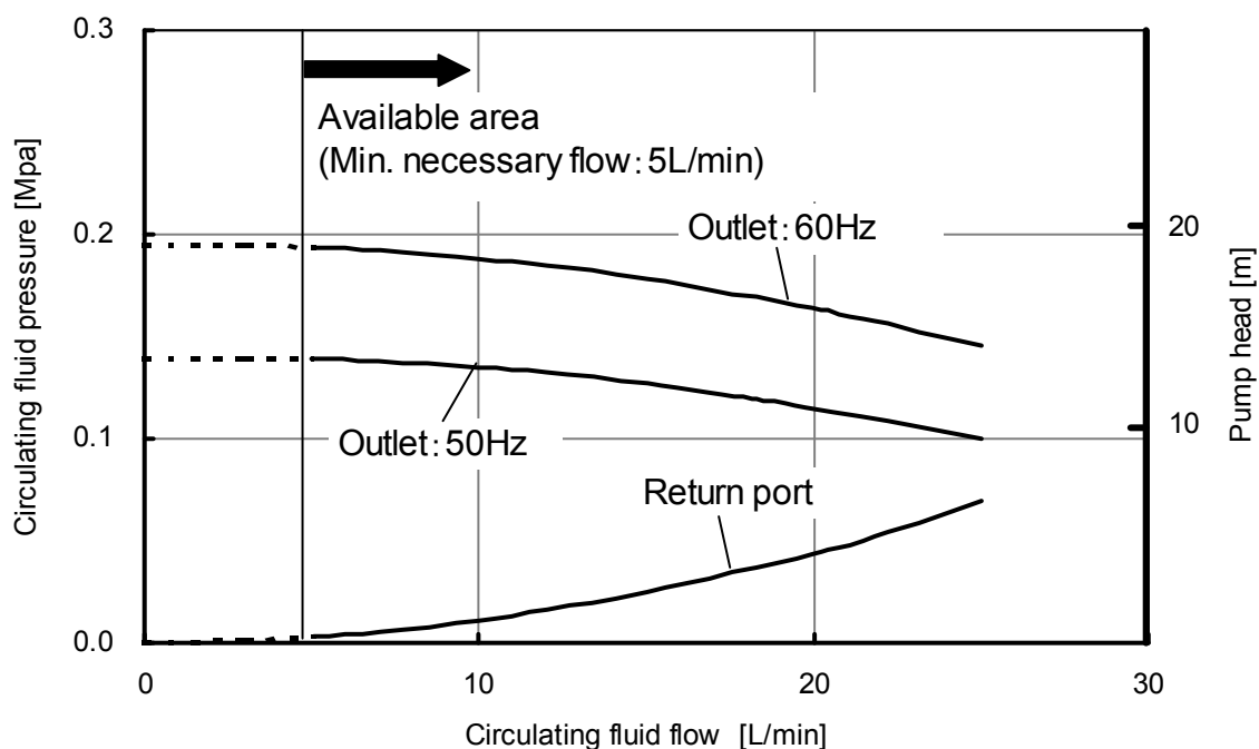
Fig. 9-14 Pump capacity(HRS012-**-10-(BJM), HRS018-**-10-(BJM))
