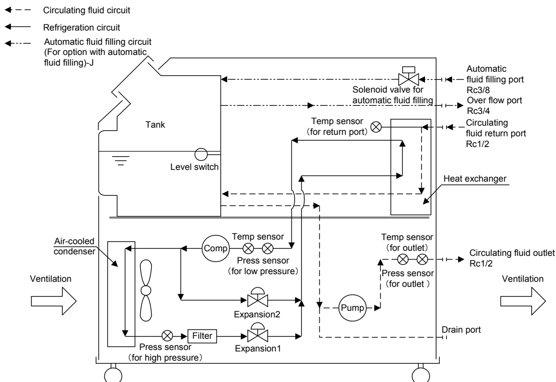
Fig. 9-2 Flow Chart(HRS012-A*-0, HRS018-A*-0, HRS024-A*-20)
