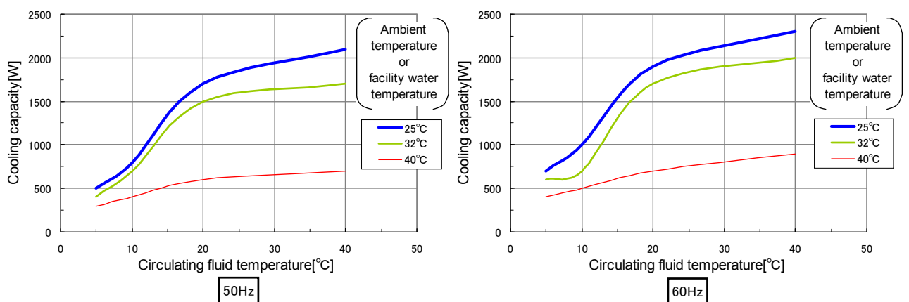
Fig. 9-7 Cooling capacity(HRS018-**-20)
