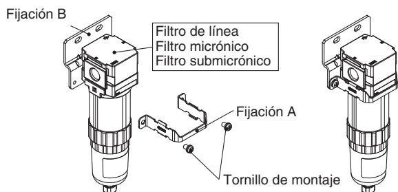
Vista de montaje con fijaciones
