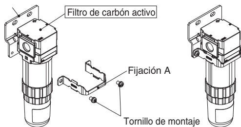
Vista de montaje con fijaciones
