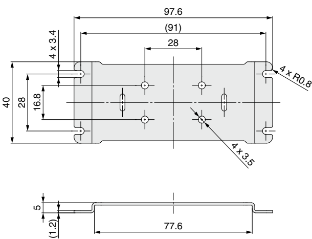
Bracket (ZS-53-G)
