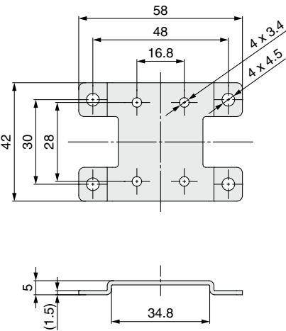
Bracket (ZS-40-L)
