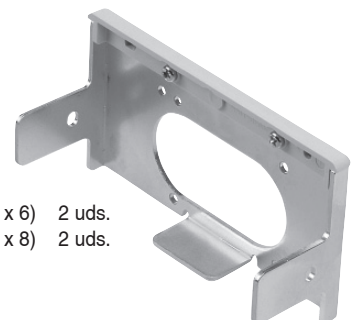
EX600-ZMV2 (Para las series SY y JSY)
