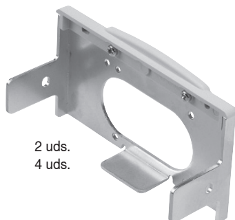
EX600-ZMV1 (Para las series SV, S0700 y VQC)
