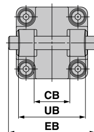
Double clevis (D)
