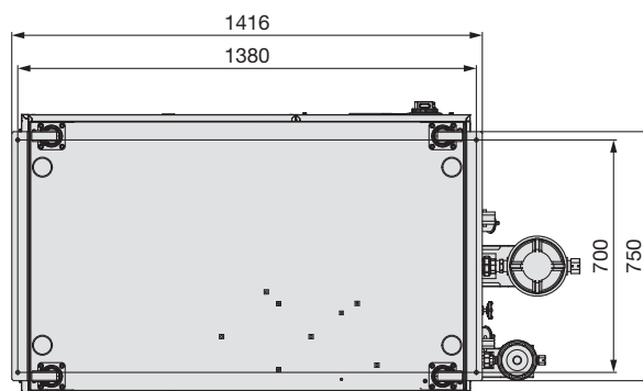
Posición de montaje de perno de anclaje (vista A)
