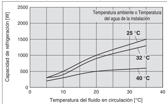
HRR018-A- -10 / -20 , HRR018-W- -10 / -20 [50 Hz]
