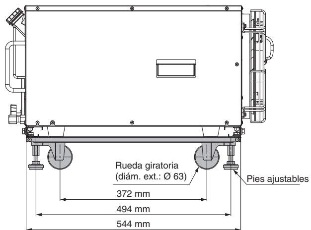
Vista de montaje (HRR012/018-A-□)
