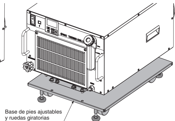
Vista de montaje (HRR012/018-A-□)
