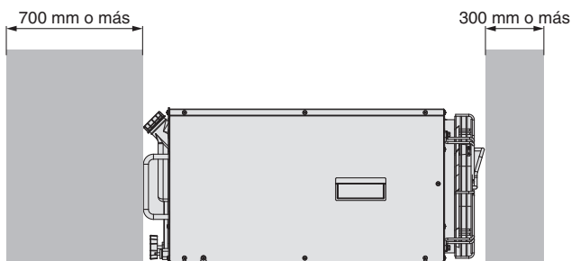
Lado frontal del producto
