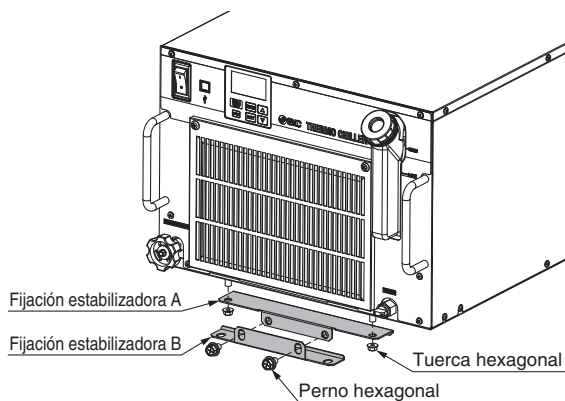
Vista de montaje (HRR012/018-A-□)
