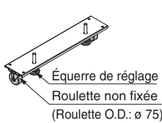
Fig. 2 Fixation de réglage de la roulette (2 pcs.)
