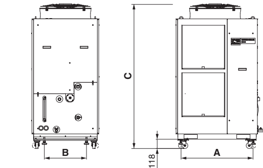
Fig. 1 Vue du montage
