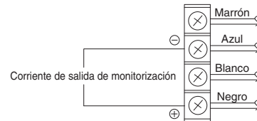
Diagrama de cableado de salida de monitorización
