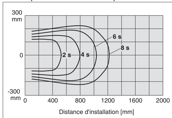
IZF21 (Nivel de caudal de aire: 10)
