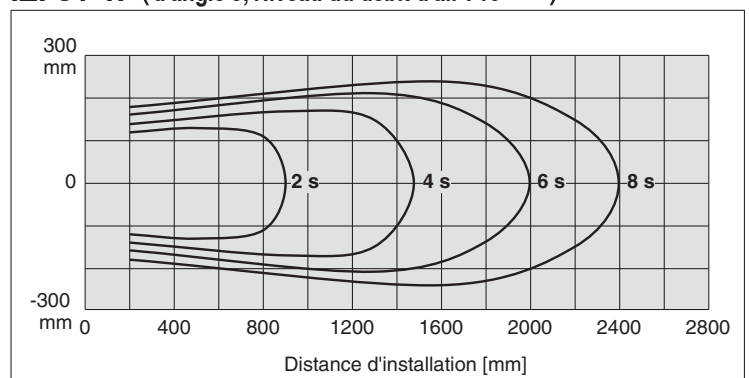
IZF31-W (Avec louvre réglable : Paramètre d'angle 5, Niveau du débit d'air : 10)
