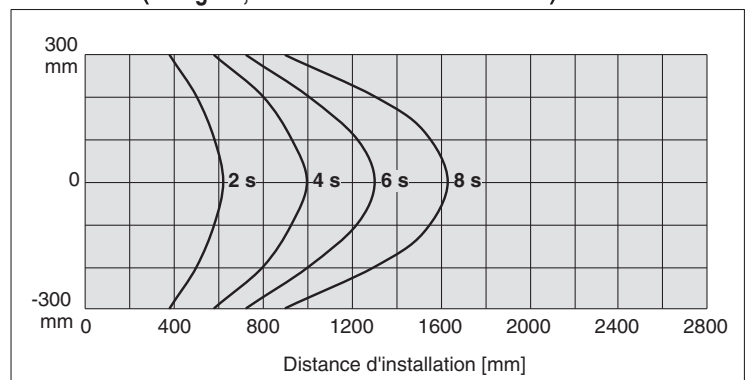
IZF31-W (Avec louvre réglable : Paramètre d'angle 1, Niveau du débit d'air : 10)
