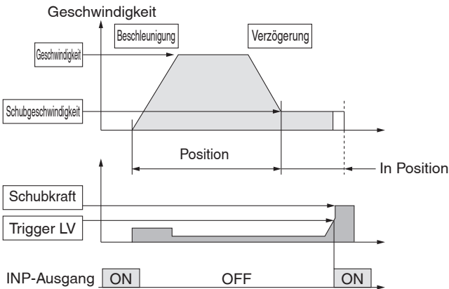
Schrittdaten (Schubbetrieb)
