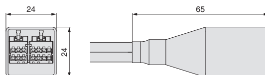
Abmessungen der Steckerabdeckung des batterielosen Absolutwertgebers
