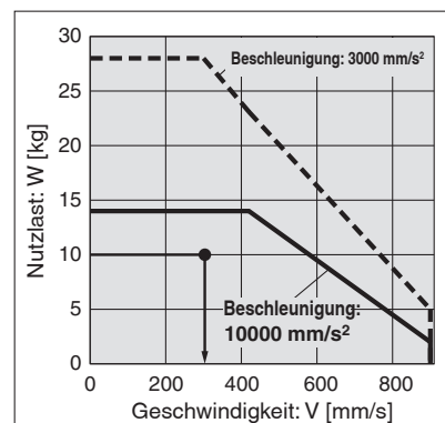
<Geschwindigkeits-Nutzlast-Diagramm> (LEFS25GA/Batterieloser Absolutwertgeber)
