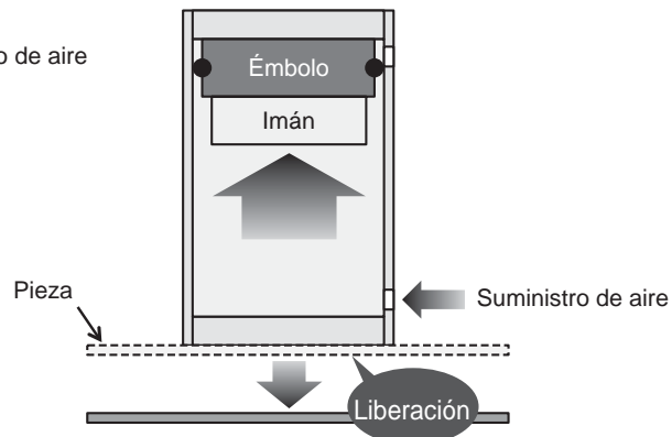
Liberación de la pieza
