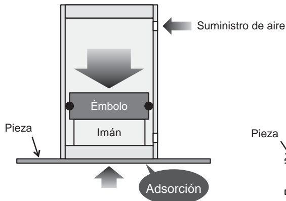
Adsorción/sujeción de la pieza
