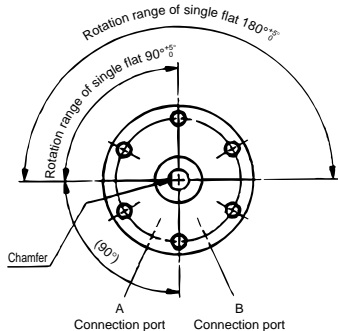
Single vane: 90°, 180°
