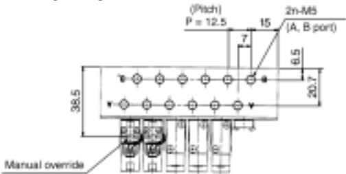
For M5
