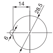
Épaisseur de la plaque VHL212W : max. 3,5
