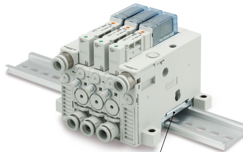
Fijación de montaje sobre rail DIN
