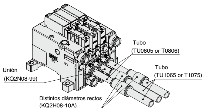
Figura. B Ejemplo de conexionado
