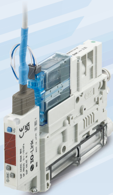
Vacuostato compatible con IO-Link La función de ahorro energético se puede activar y desactivar ajustando los parámetros.
