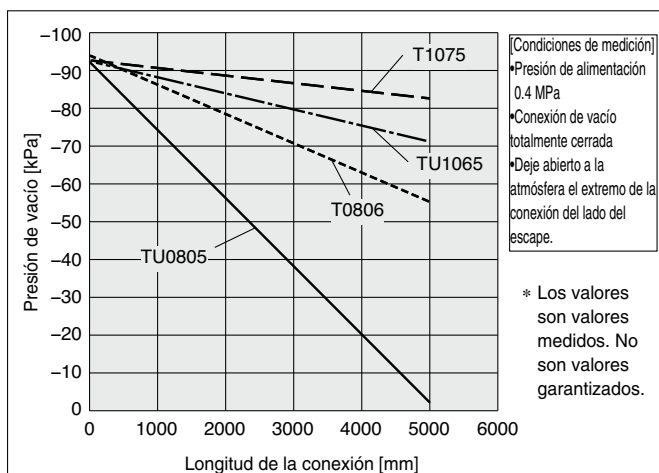
Figura. A. Presión de vacío para conexionado (ZK2□15)
