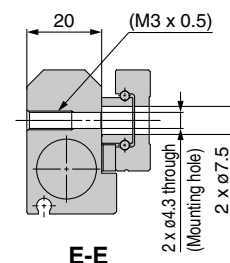
E-E
